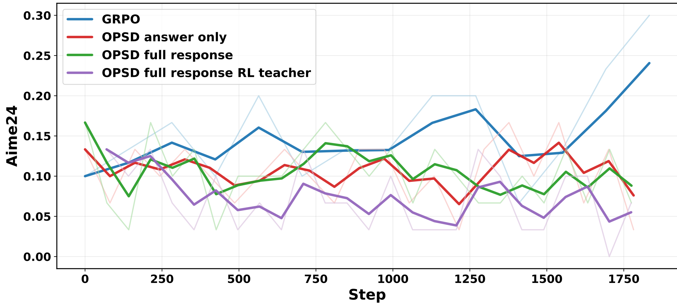
eval/aime24
